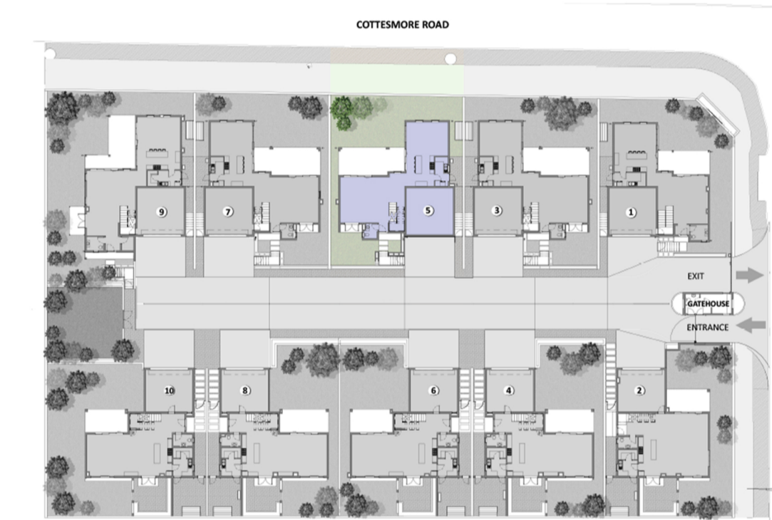
SITE PLAN 1:500
