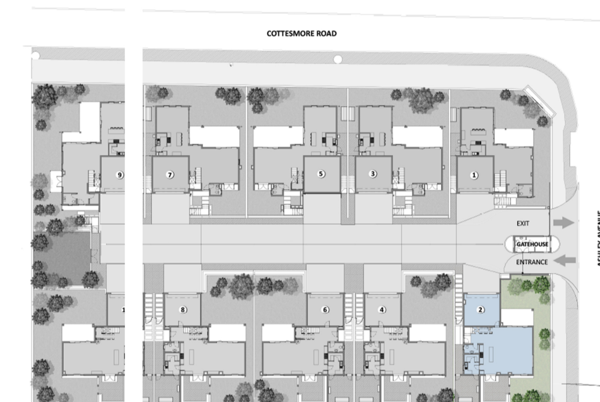
SITE PLAN 1:250
